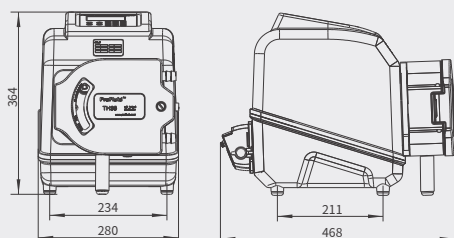
外形尺寸图
