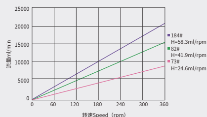
TH35流量曲线图
