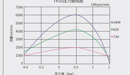
TH35压力曲线图
