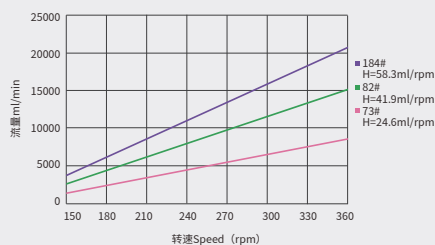
TH35流量曲线图
