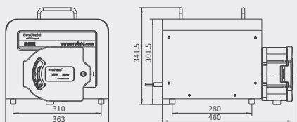
外形尺寸图
