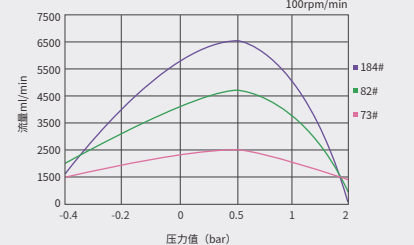
TH35压力曲线图
