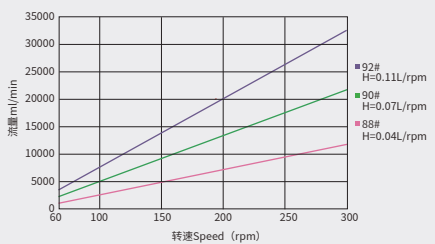
XC45流量曲线图
