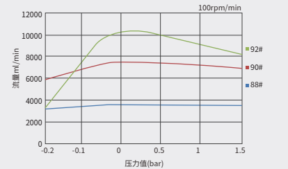
XC45压力曲线图
