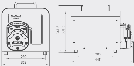
外形尺寸图
